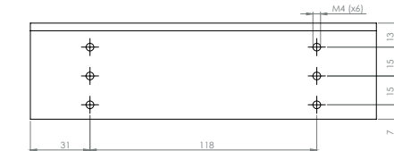
„L” konzol
