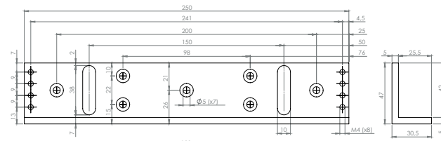
„L” konzol
