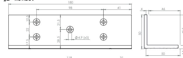
„Z” konzol
